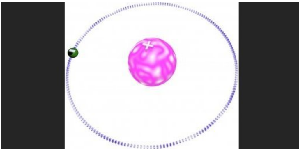
Toli nuo teigiamai įkrauto jono skriejantis elektronas Rydbergo atome
