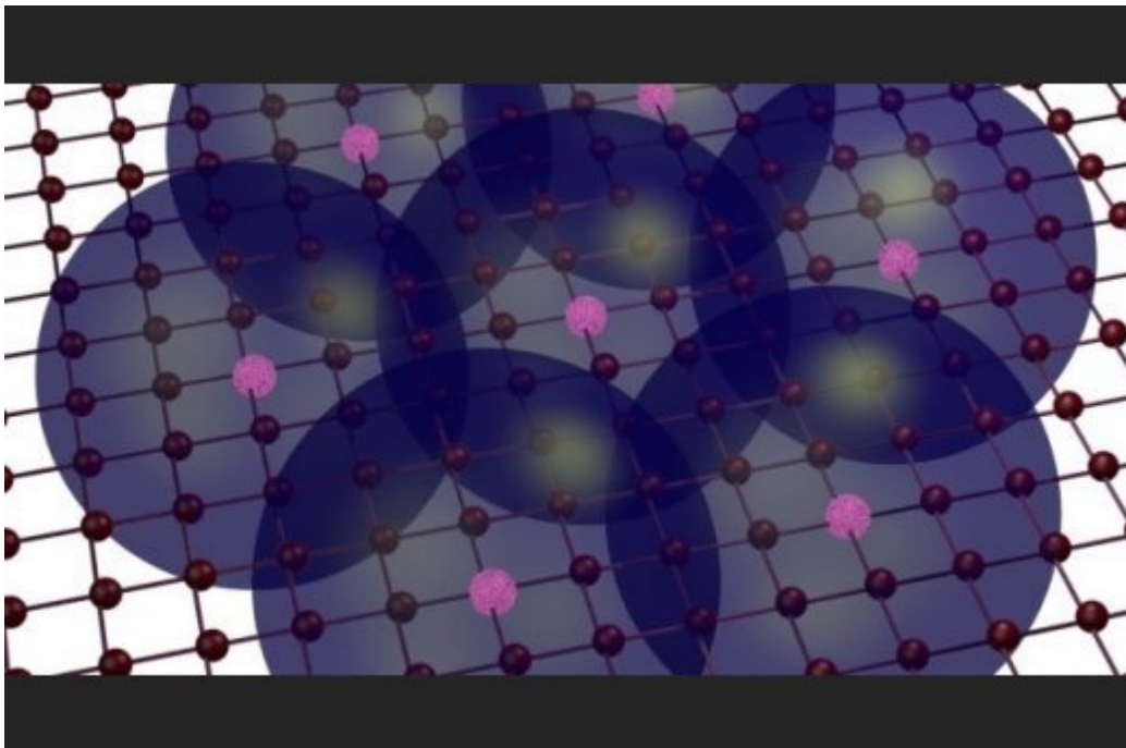
Persiklojantys skirtingų Rydbergo atomų elektronų debesėliai
